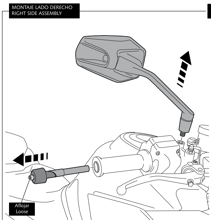
MONTAJE LADO DERECHO RIGHT SIDE ASSEMBLY
